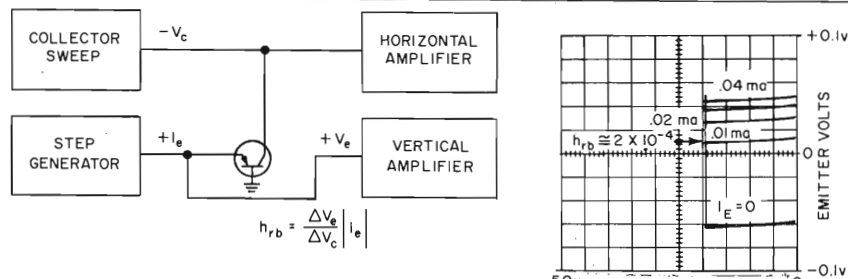
(D) VOLTAGE FEEDBACK RATIO, h_{ib} , h_{re}
